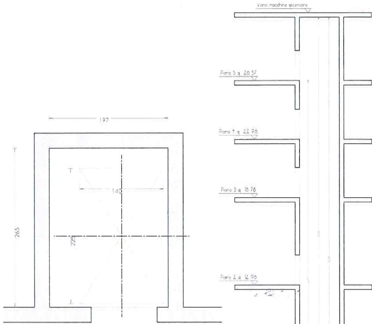
Pianta Scala 1/20
